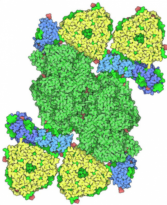
figure 1 - le supercomplexe du photosystème ii du pois le photosystème est représenté en vert foncé, l'antenne collectrice lhci en jaune et les complexes d'antennes mineurs en bleu. les différents cofacteurs sont représentés en vert clair et en rouge.
