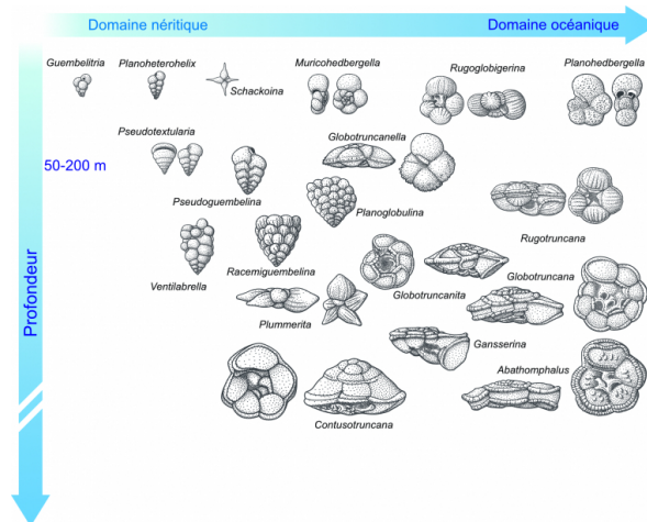
figure 1 - distribution dans la tranche d'eau des principaux genres de foraminifères planctoniques du crétacé terminal aux basses latitudes
