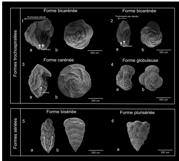
figure 2 - les différentes architectures de test des foraminifères planctoniques du crétacé supérieur micrographies obtenues au microscope électronique à balayage. les espèces figurées proviennent du maastrichtien supérieur de la coupe type de bidart (pyrénées atlantiques, france). spécimens 1 à 3 : globotruncanidae (formes trochospirales) illustrés sur le profil (a) et la face spirale (b). 1. contusotruncana contusa . 2. globotruncana arca . 3. globotruncanita stuarti (– 15 cm sous la limite crétacé-paléogène). spécimen 4. rugoglobigerinidae (forme trochospirale), rugoglobigerina rugosa (– 180 cm sous la limite crétacé-paléogène). spécimens 5 à 6 : heterohelicidae (formes sérées). 5. pseudotextularia elegans . 6. racemiguembelina fructicosa (– 180 cm sous la limite crétacé-paléogène).
