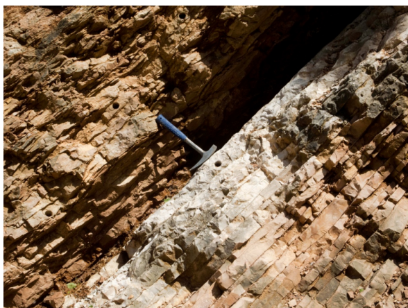
figure 4 - la limite crétacé-paléogène affleurant dans la vallée de la contessa, région de gubbio (italie)
