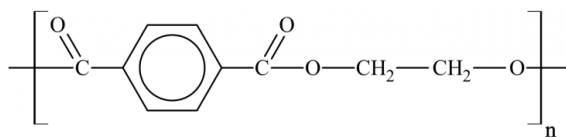
figure 1 - formule développée du pet ou polytéréphtalate d'éthylène, un plastique
