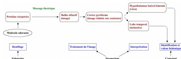
figure 4 - les voies de l'odorat
