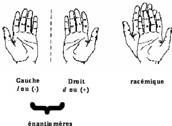
figure 2 - illustration de la notion de chiralité les mains sont des objets chiraux. un mélange de deux énantiomères, molécules images l'une de l'autre dans un miroir plan mais non superposables, est dit racémique.
