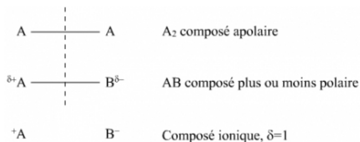
figure 1 - polarité de molécules diatomiques
