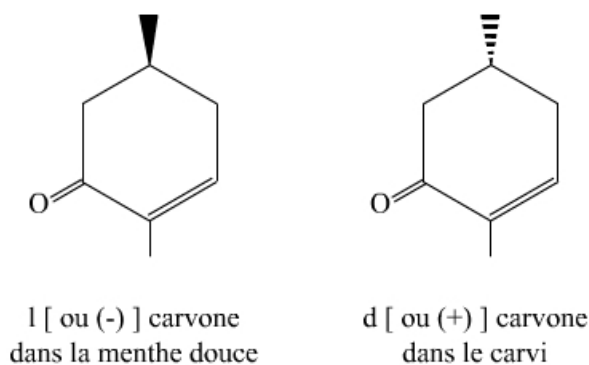
figure 3 - la carvone selon l'énantiomère considéré, la sensation perçue sera différente bien qu'il s'agisse de la même molécule.
