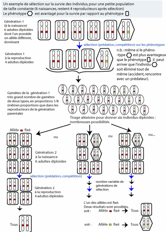
figure 3 - un exemple de sélection d'un allèle
