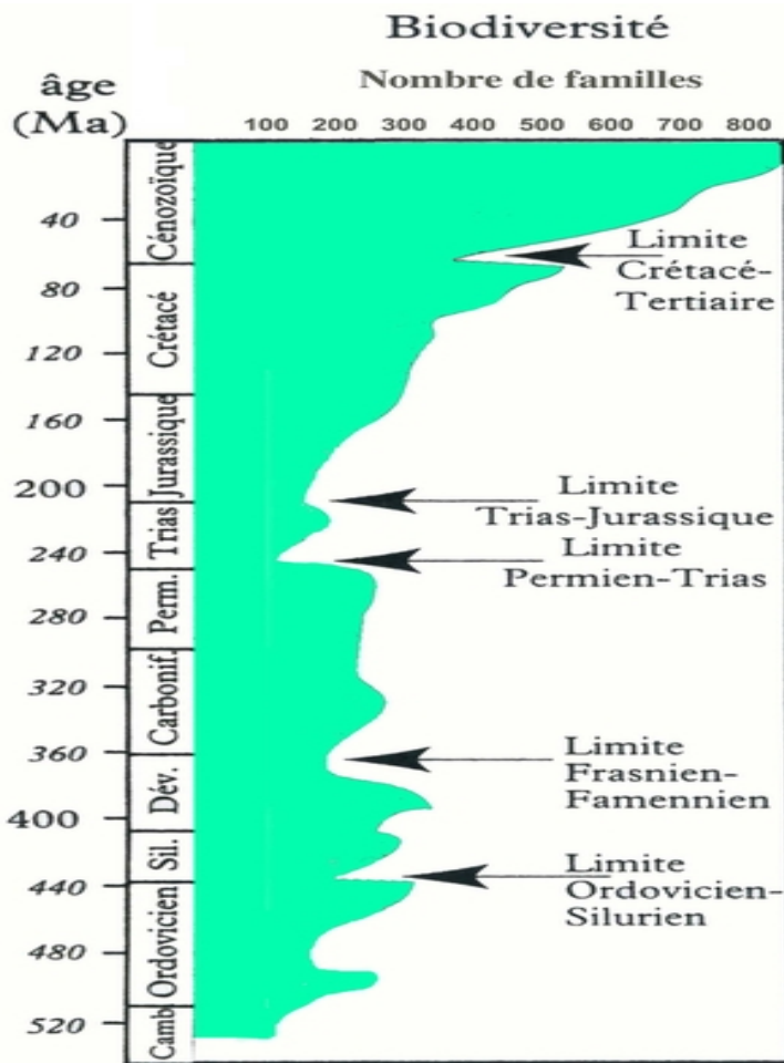
figure 9 - les grandes extinctions des temps géologiques les limites sont mises en évidences par la diminution rapide du nombre de familles.
