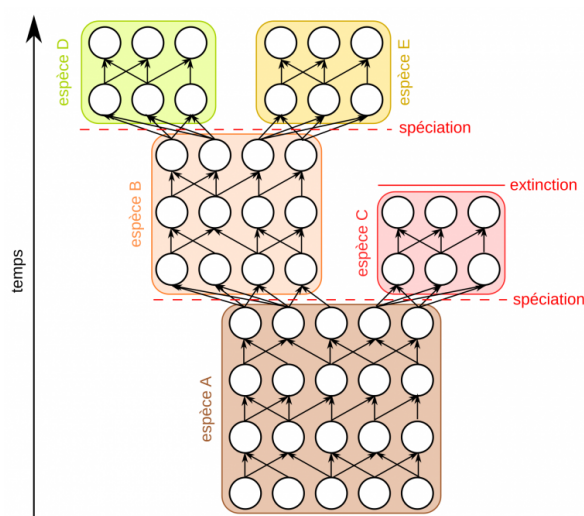
figure 6 - évolution des espèces et spéciations chaque rond représente un individu. les flèches représentent les liens de parenté entre individus. si deux populations ne peuvent plus se reproduire, on considère qu'il y a formation de deux nouvelles espèces.
