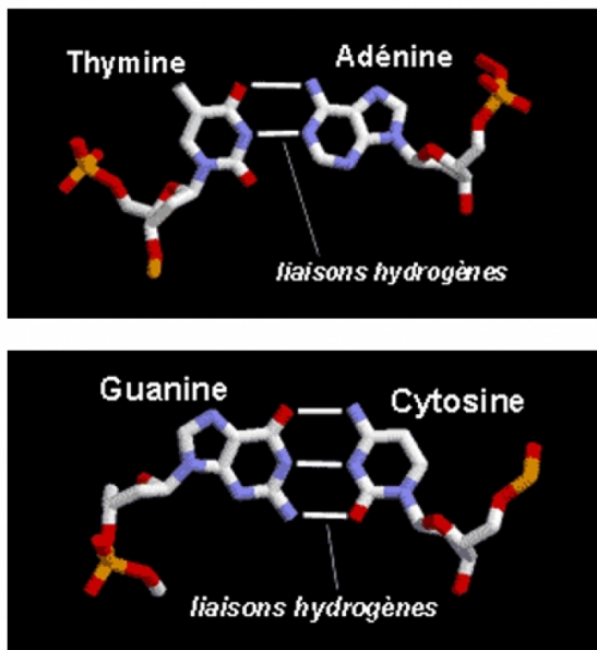
figure 3 - les bases azotées peuvent s'associer deux à deux par des liaisons hydrogènes.
