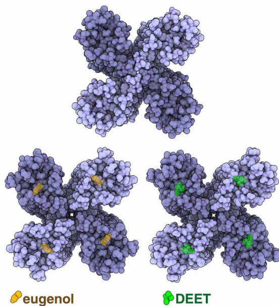
figure 2 - le canal or5 peut fixer différentes substances comme l'eugénol et le deet le canal constitué de quatre monomères or5, représenté fermé en haut de la figure (entrée pdb 7lic ), s'ouvre après avoir fixé différentes molécules odorantes, comme l'eugénol (en orange, entrée pdb 7lid ) et le deet (en vert, entrée pdb 7lig ).
