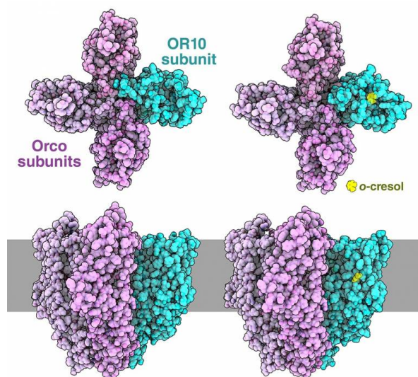
figure 1 - les récepteurs olfactifs des insectes en configuration fermée ou ouverte avec du o-crésol les récepteurs olfactifs des insectes sont des canaux ioniques constitués de quatre sous-unités. sur le canal représenté ici (entrées pdb 8v00 et 8v02 ), les sous-unités orco sont représentées en rose, tandis que la sous-unité or est en turquoise. sur la droite, le récepteur est représenté en configuration ouverte après fixation d'un ligand, l'o-crésol (en jaune). en haut : vue du dessus ; en bas : vue de profil, avec le récepteur inséré dans la membrane plasmique (en gris)
