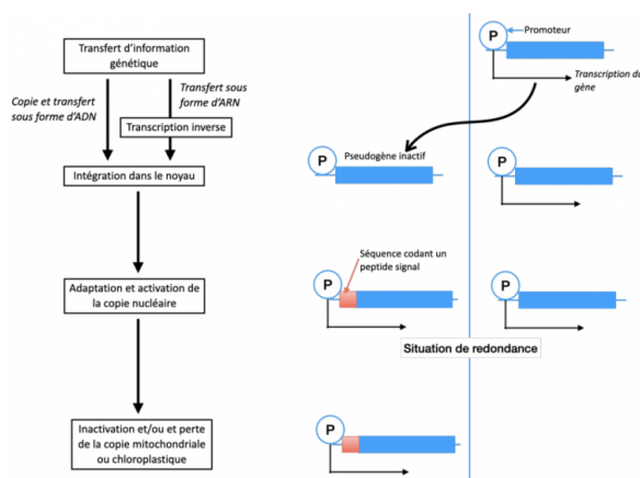
figure 15 - mécanisme de transfert horizontal de gènes des organites vers le noyau
