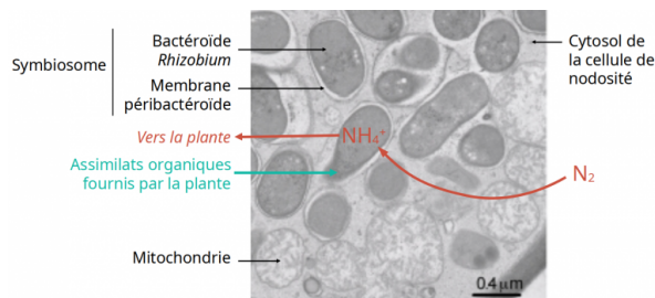
figure 2 - structure et fonctionnement d'une symbiose entre une bactérie du genre rhizobium et une fabacée, le lotier lotus japonicus les bactéries sont incluses, sous forme de bactéroïdes, dans la membrane pér bactéroïde, d'origine végétale. l'ensemble se comporte comme un organe, le symbiosome, spécialisé dans la fixation du diazote venant de l'atmosphère. selon les espèces hôtes, chaque symbiosome peut contenir une seule ou plusieurs bactéries, soit par fusion de plusieurs symbiosomes, soit par division bactérienne [2b].
