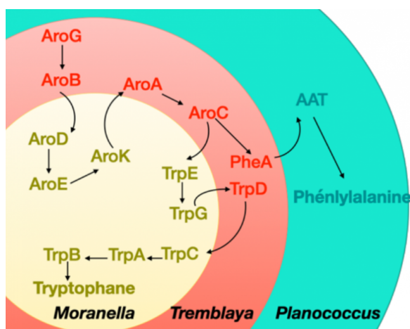
figure 5 - répartition des voies de biosynthèse du tryptophane et de la phénylalanine entre les trois partenaires symbiotiques chez la cochenille farineuse les intermédiaires des voies de biosynthèse sont indiqués par leurs initiales à 3 lettres.
