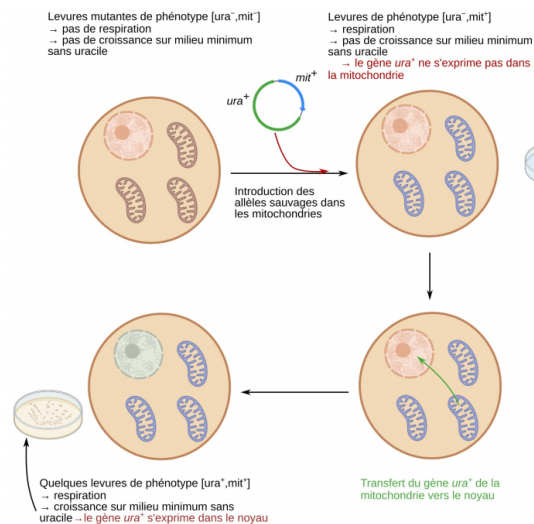
figure 14 - mise en évidence expérimentale d'un transfert de gènes entre mitochondrie et noyau chez la levure saccharomyces cerevisiae
