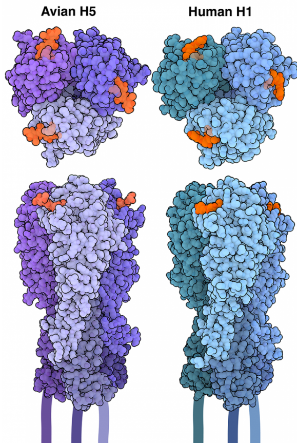
figure 1 - les hémagglutinines h5 et h1 liées à des analogues d'acides sialiques les trimères d'hémagglutinine liés à des analogues de récepteurs d'acides sialiques (en orange) sont représentés en vue de dessus et de côté. l'hémagglutinine h5 de la grippe aviaire est représentée en violet et l'hémagglutinine h1 de la grippe humaine est représentée en bleu.
