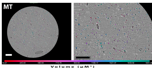
figure 1 - microtomogramme haute résolution d'échantillon de couche interne de l'os pétreux avec analyse des volumes des lacunes ostéocytaires les couleurs donnent une indication qualitative des volumes des lacunes. barres d'échelle = 100 µm.
