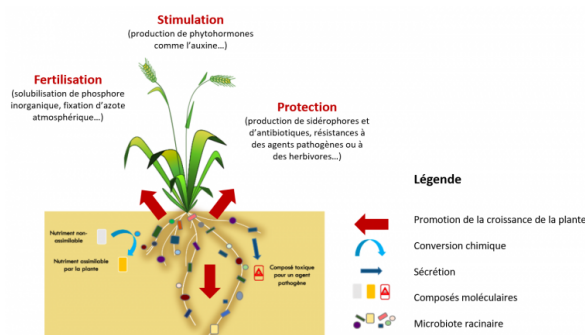
figure 4 - les fonctions du microbiote racinaire dans la survie des plantes la croissance de la plante est soutenue par trois fonctions portées par son microbiote racinaire que sont la fertilisation, la stimulation de la croissance et la protection.
