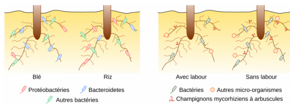
figure 2 - variation de la composition du microbiote en fonction de l'espèce de plante et des techniques de culture à gauche. effet du géotype de la plante (riz ou blé) sur le microbiote bactérien racinaire. à droite. effet d'un facteur environnemental (la pratique du labour) sur le microbiote bactérien et fongique racinaire.
