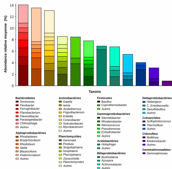
figure 3 - abondance relative des bactéries et archées des sols de france métropolitaine abondances relatives moyennes (en ordonnée) des 12 phyla et 47 genres principaux de bactéries et archées (en abscisse) retrouvés dans 2173 échantillons de sols répartis sur l'ensemble de la france métropolitaine. les catégorie « autres » correspond à la somme de tous les genres de chaque phylum représentant moins de 0,5% des séquences d'adn servant à l'identification des micro-organismes.
