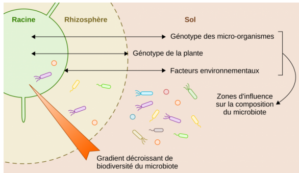
figure 1 - le microbiote racinaire des plantes schéma d'une coupe transversale de racine de plante présentant les compartiments colonisés par des microbiotes spécifiques (racine, rhizosphère et sol), le gradient de biodiversité du microbiote et les facteurs influençant la composition du microbiote dans chaque compartiment : génotype des micro-organismes, génotype de la plante, environnement de la plante.
