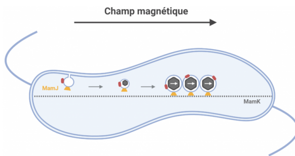
figure 5 - la biogénèse des magnétosomes chez les bactéries magnétotactiques plusieurs protéines sont recrutées au niveau de la membrane plasmique et permettent son invagination et donc la formation de vésicules. d'autres protéines spécialisées (en rouge) sont chargées de transporter le fer dans le lumen du magnétosome en formation créant des conditions chimiques propices à la nucléation et la croissance de cristaux de fer. l'alignement des vésicules entre elles est, entre autres, assuré par l'interaction entre les protéines spécialisées mamj (en jaune) et le cytosquelette composé de mamk (ligne pointillée) similaire au cytosquelette d'actine. en s'alignant, la chaîne de magnétosomes forme un dipôle magnétique permettant à la cellule de s'aligner le long des lignes de champ magnétique. schéma réalisé à l'aide de biorender .
