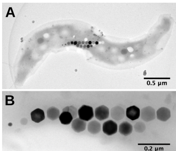
figure 2 - le magnétosome : un organite propre aux bactéries magnétotactiques bactérie magnétotactique (a) observée au microscope électronique à transmission. les magnétosomes (b) s'alignent le long de la bactérie selon son axe de motilité. leur taille ne permet de les observer qu'en microscopie électronique où ils apparaissent denses aux électrons.
