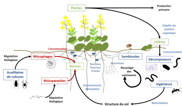
figure 2 - impacts directs et indirects de la faune du sol sur la production primaire dans les agroécosystèmes les boîtes indiquent les différents groupes fonctionnels impliqués dans les services écosystémiques (en noir), les éléments bleu représentent les processus à effets positifs sur les plantes, les éléments en rouge représentent les processus à effets négatifs.
