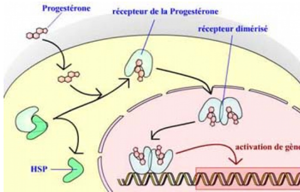
figure 3 - schéma du mode d'action de la progestérone auteur(s)/autrice(s) : david germanaud, gilles furelaud licence : pas de licence spécifique (droits par défaut)
