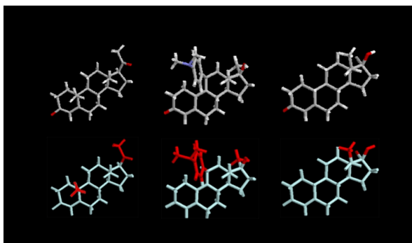
figure 1 - structures tridimensionnelles de la progestérone, de la mifépristone (ru-486) et du lévonorgestrel de gauche à droite : molécule de progestérone, molécule de mifépristone et molécule de lévonorgestrel. trois schémas du haut: en gris le squelette de carbone, en blanc les atomes d'hydrogène, en rouge les atomes d'oxygène et en bleu les atomes d'azote. trois schémas du bas: en gris-bleu le noyau stérol et en rouge les autres groupements.
