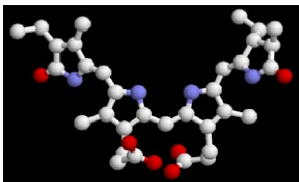
figure 13 - formule d'une phycobiline l'exemple présenté ici est la phycocyanobiline, représentée sans la protéine qui l'accompagne normalement.
