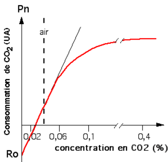
figure 19 - influence de la concentration en \text{CO}_2 de l'air sur la consommation en \text{CO}_2 d'une plante verte
