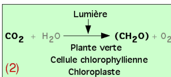
figure 9 - équation bilan dédiée de ces expériences : équation (2)
