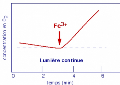
figure 23 - nécessité d'un absorbeur d'électron pour la photosynthèse en absence de \text{CO}_2 , les chloroplastes sont capables de libérer du dioxygène, à condition qu'un accepteur d'électron ( \text{Fe}^{3+} ) soit présent dans le milieu.
