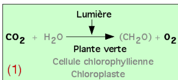
figure 7 - équation bilan de la photosynthèse : équation (1) l'expérience précédente montre qu'à la lumière, une plante verte produit de l' \text{O}_2 si du \text{CO}_2 lui est fourni. cette constatation n'implique aucune relation chimique entre le \text{CO}_2 et l' \text{O}_2 .
