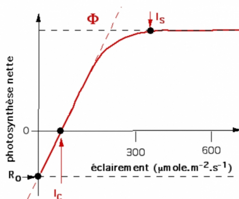
figure 17 - influence de l'éclairement sur la photosynthèse nette
