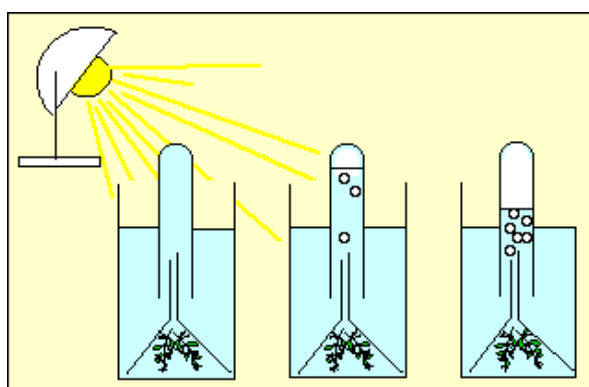
figure 6 - expérience de dégagement de dioxygène par une élodée à la lumière les trois expériences sont réalisées dans : (a) de l'eau distillée ; (b) de l'eau du robinet ; (c) de l'eau additionnée d'hydrogénocarbonate à 1 %. c'est en (c) que la production d'oxygène est la plus importante.
