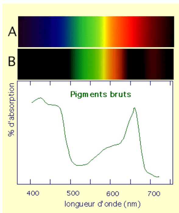
figure 14 - spectre d'absorption des pigments bruts extraits à partir d'une feuille a : spectre lumineux en absence de pigments. b : spectre lumineux en présence de pigments. on note que l'absorption maximale se réalise dans le bleu et dans le rouge.
