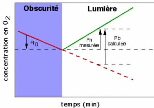
figure 16 - évolution de la concentration en dioxygène à l'obscurité et à la lumière lors de la photosynthèse pb = pn - ro
