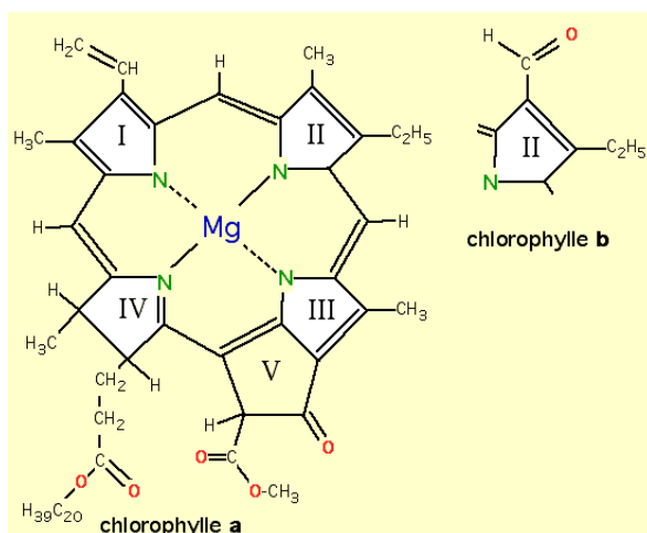
figure 11 - formules des chlorophylles a et b les chlorophylles diffèrent par les substituants des groupements pyrroles. le phytol n'est pas détaillé ici. légende : i, ii, iii, iv = groupements pyrroles et v = cycle supplémentaire.
