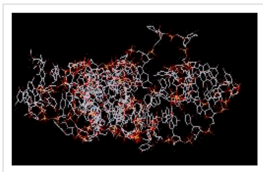
figure 2 : sous unité d'hémoglobine (eric martz)
