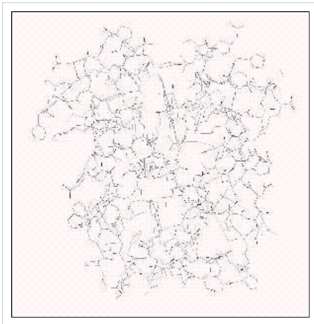
figure 3 : différentes représentations d'une sous-unité de l'hémoglobine
